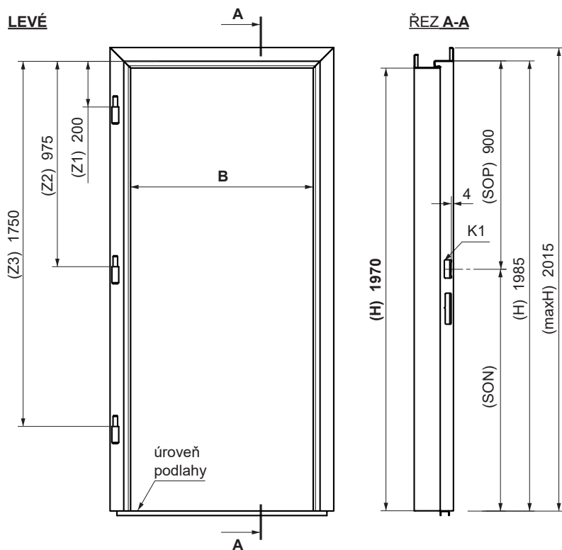
ŘEZ PROFILU ZÁRUBNĚ ČÁSTEČNĚ SKRYTÉ TYP HSS
