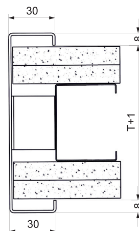
TVAR PROFILU
